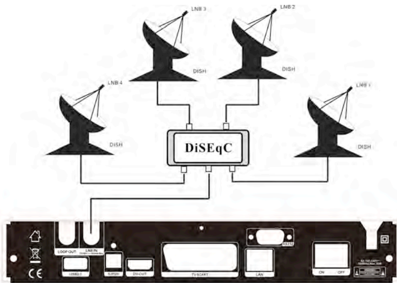
Abbildung 7. Verbindung mit LNB mit Hilfe von DiSEqC
